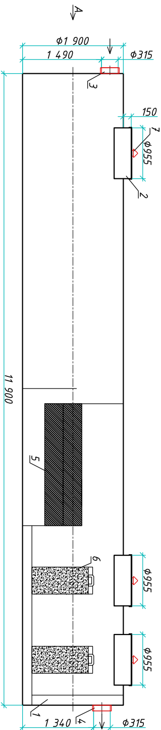
Разрез 1-1
